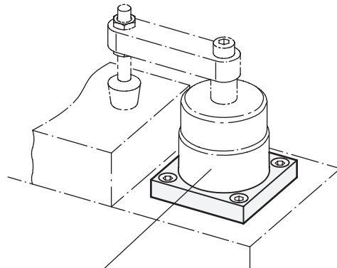
摆动夹具 GN 876
